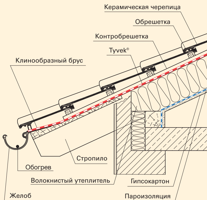
Рис. 5 Отвес
