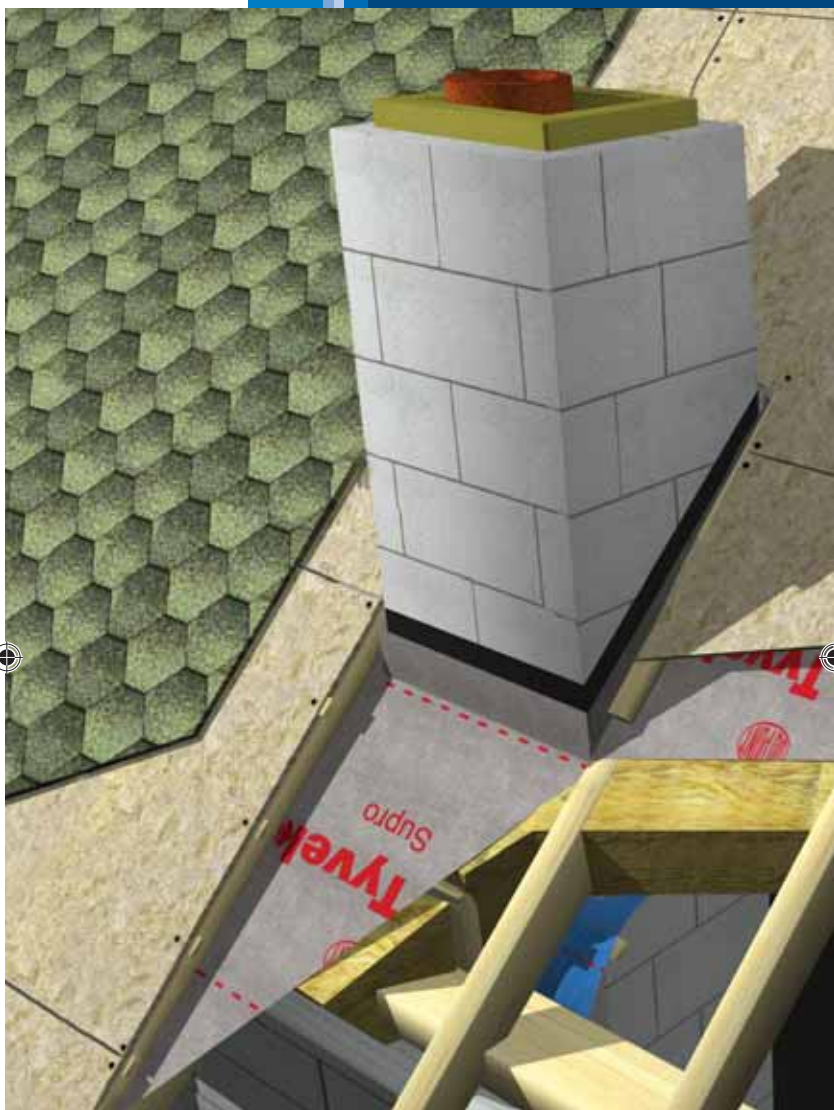
Рис. 4 Дымоход и мансардное окно
