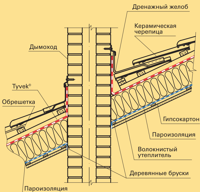
Рис. 3 Дымоход
