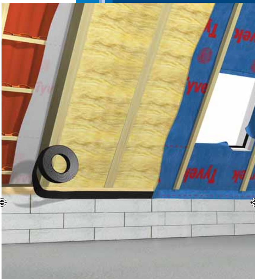
Рис. 10 Монтаж пароизоляции
