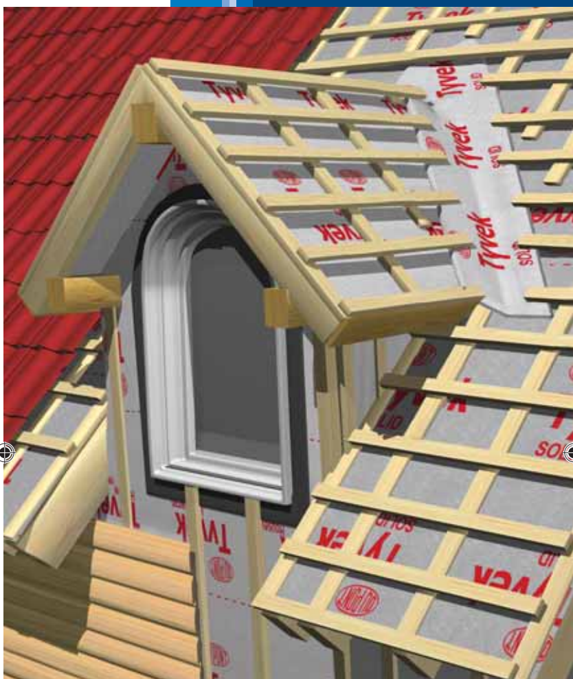
Рис. 1 Устройство утепленной мансарды
