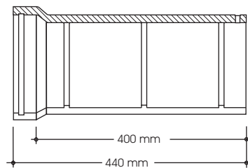
Längsschnitte
