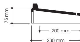
Längsschnitt
